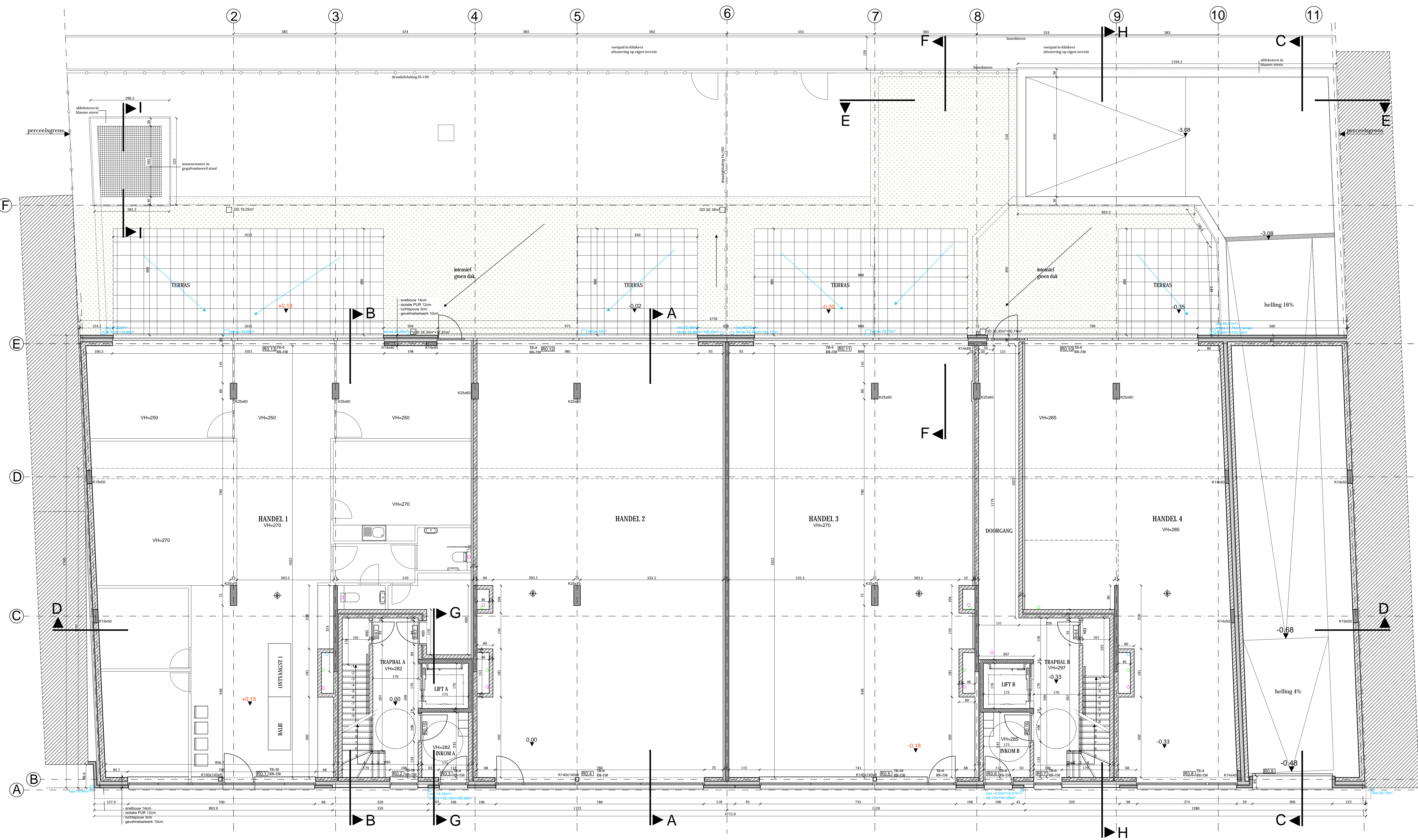
GELIJKVLOERSPLAN schaal 1/50
