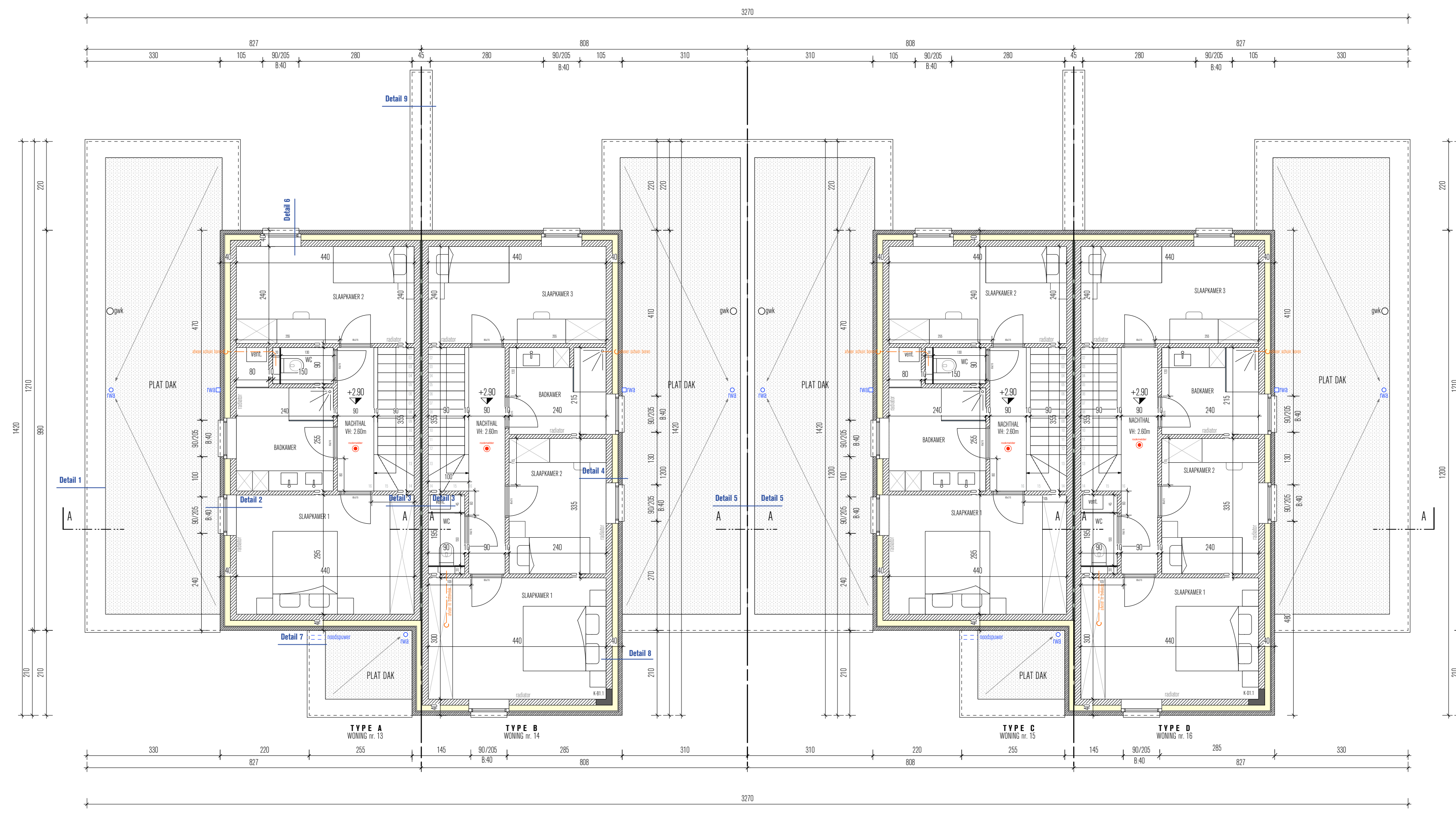
Verdieping 1 BLOK A
